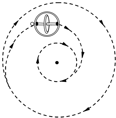
Fig. 4.23 Gyro illustrates Bohr atom!
