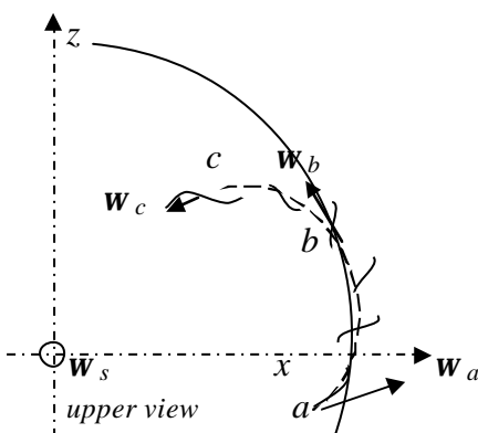
fig. 2.2 : Solar protuberance.
